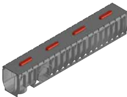
W&H - RECYFIX sportsleufgoot (NW 100 mm), type SUPER, L x B x H 1000 x 160 x 196 mm, 6,4 kg. Art. nr. WH7650
