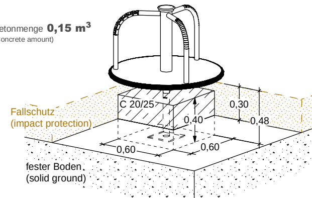
Erdanker für bauseitiges Betonfundament (Ground anchor for concrete foundation)
