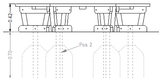
Halbe Sechseck-Bank ohne Lehne (Innen-Ø X = 0,80 m)
