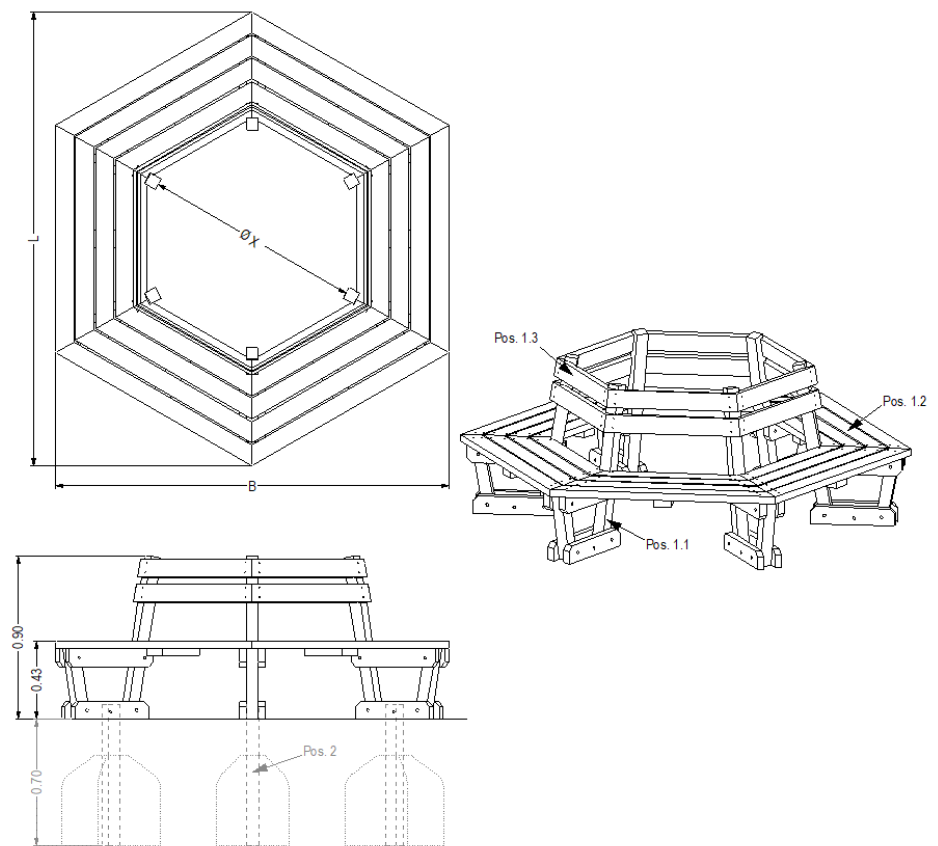
Sechseck-Bank mit Lehne (Innen-Ø X = 0,80 m | 1,20 m)
