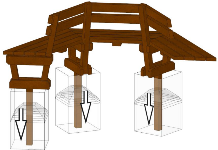
Abbildung Sechseck-Bank mit Lehne
