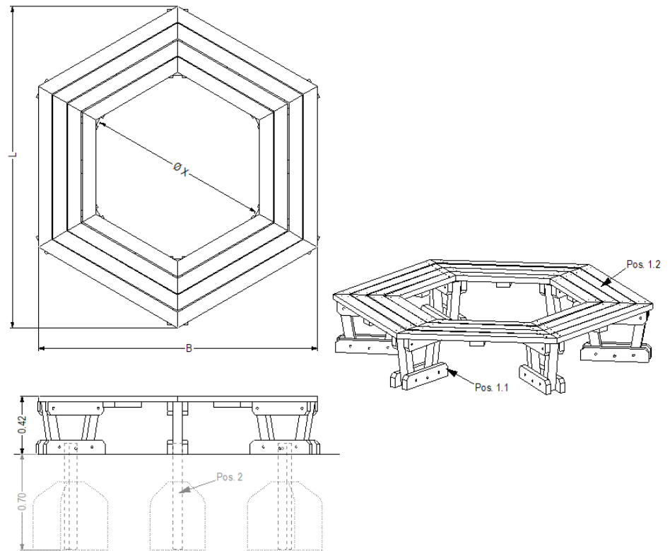
Sechseck-Bank ohne Lehne (Innen-Ø X = 0,80 m | 1,20 m)
